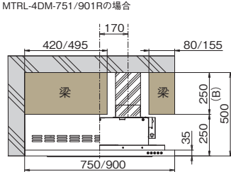
直交梁の場合
