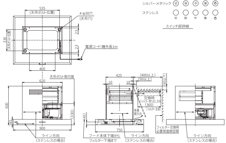
【製品寸法図】
