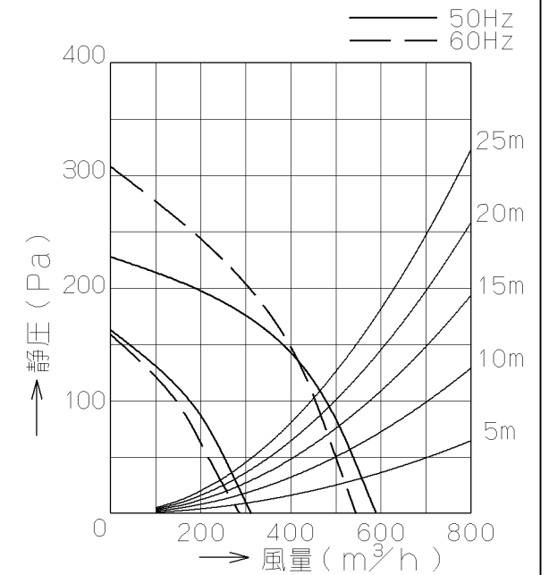
静 圧 - 風 量 曲 線
