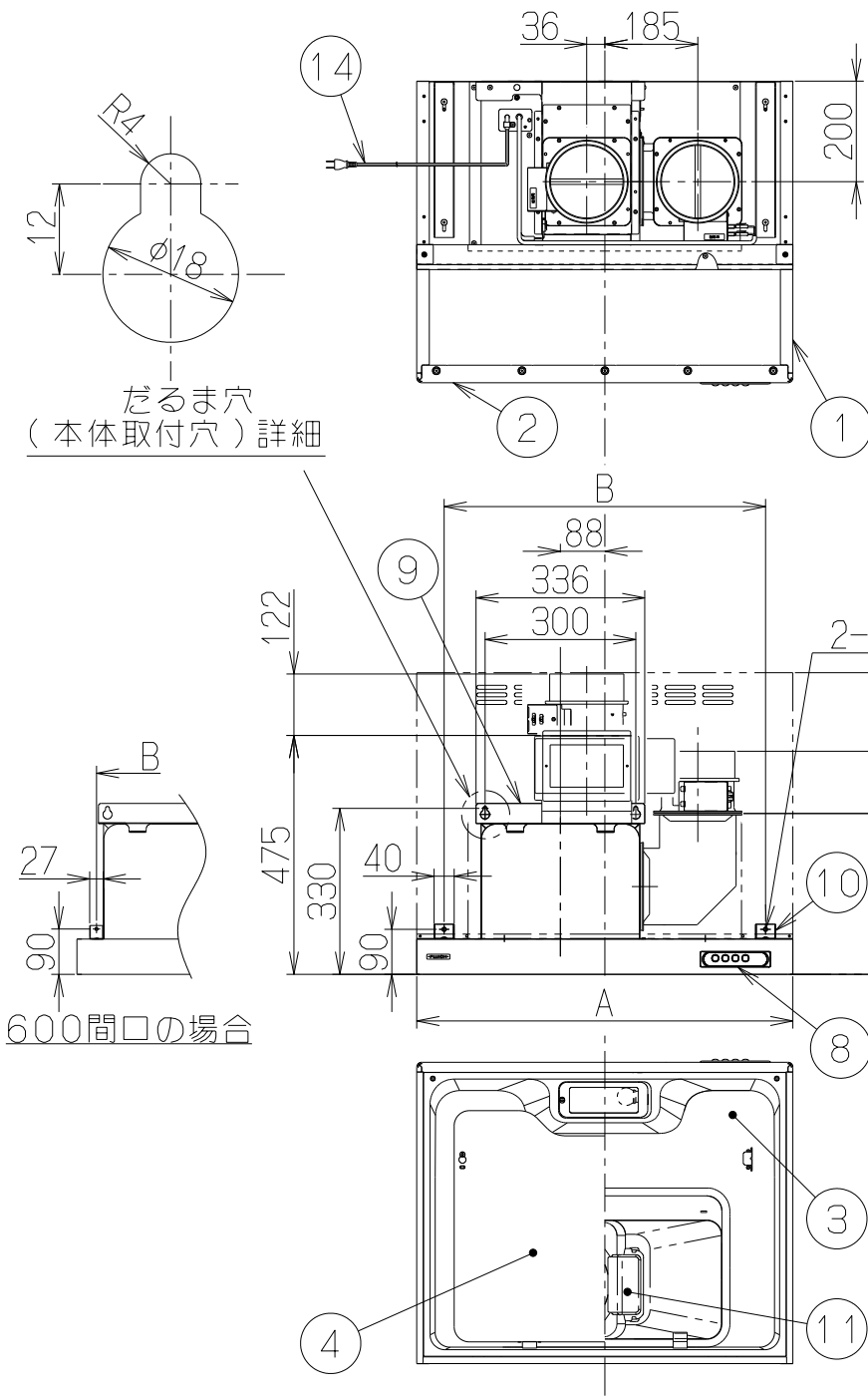
上方給気・排気の場合
