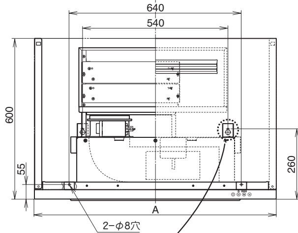
だるま穴 (本体取付穴) 詳細
