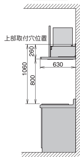
標準施工例
