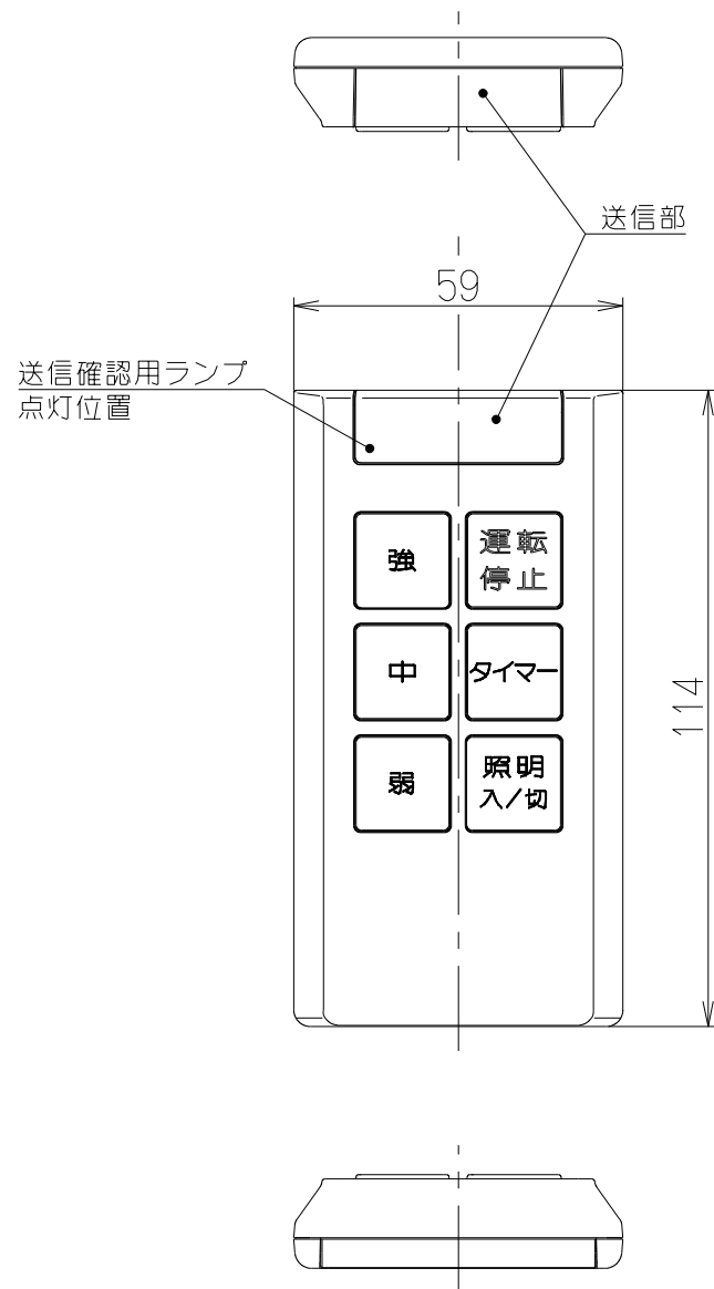
リモコン本体 (耐熱ABS)
