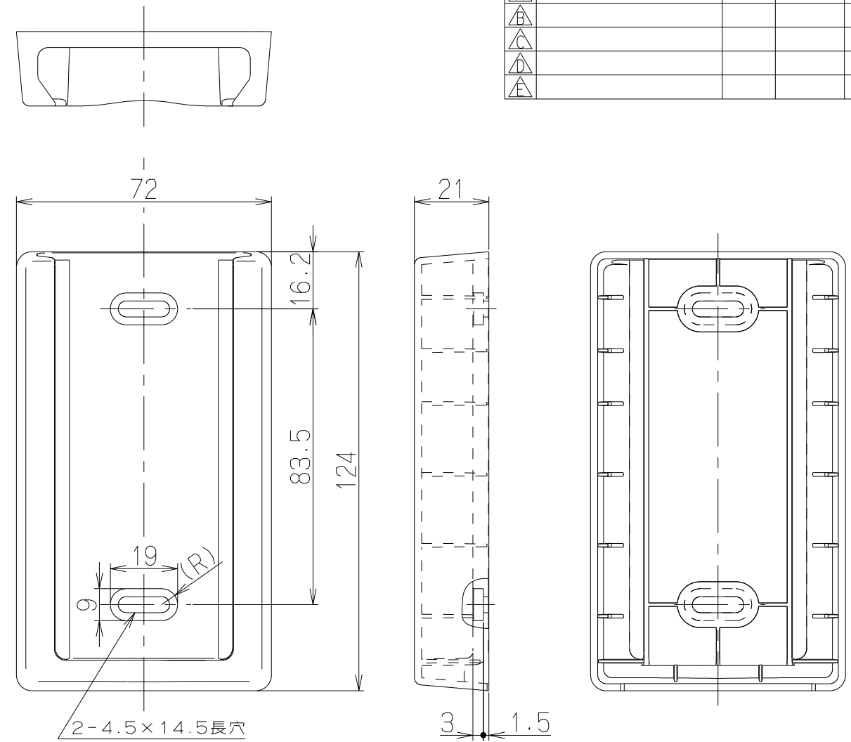
リモコンホルダー (耐熱ABS)
